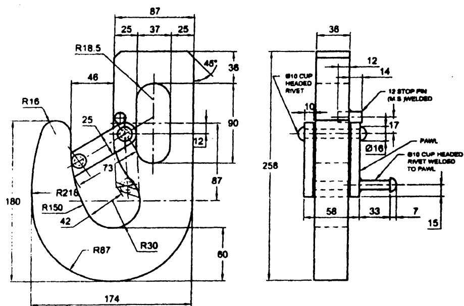
FIG. 2 HOOK
