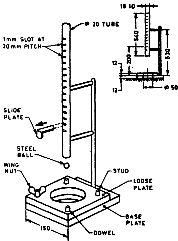
FIG. 9 SEPARATOR IMPACT Test APPARATUS
