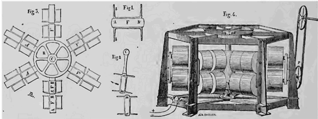
Moteur électrique, par M. Froment.
