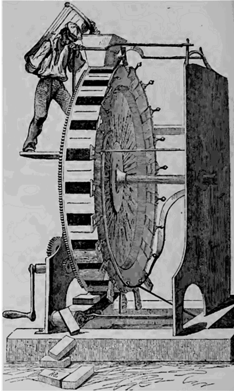
Machine à fabriquer les briques, par M. Parise.
