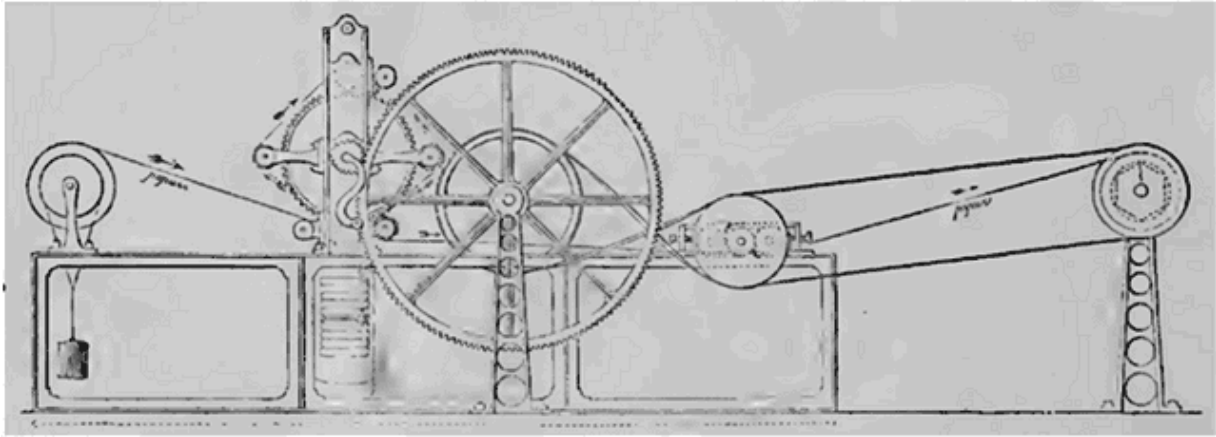
Machine à satiner le papier, par M. Callaud Belisle.
