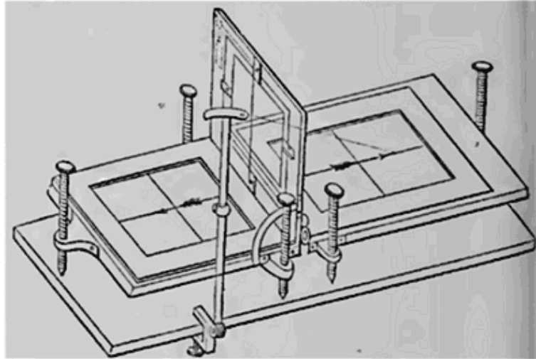
Le Calcographe, par M. Rouget de Lisle.
