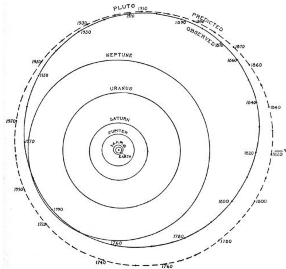
Predicted and Actual Orbits of PLUTO
