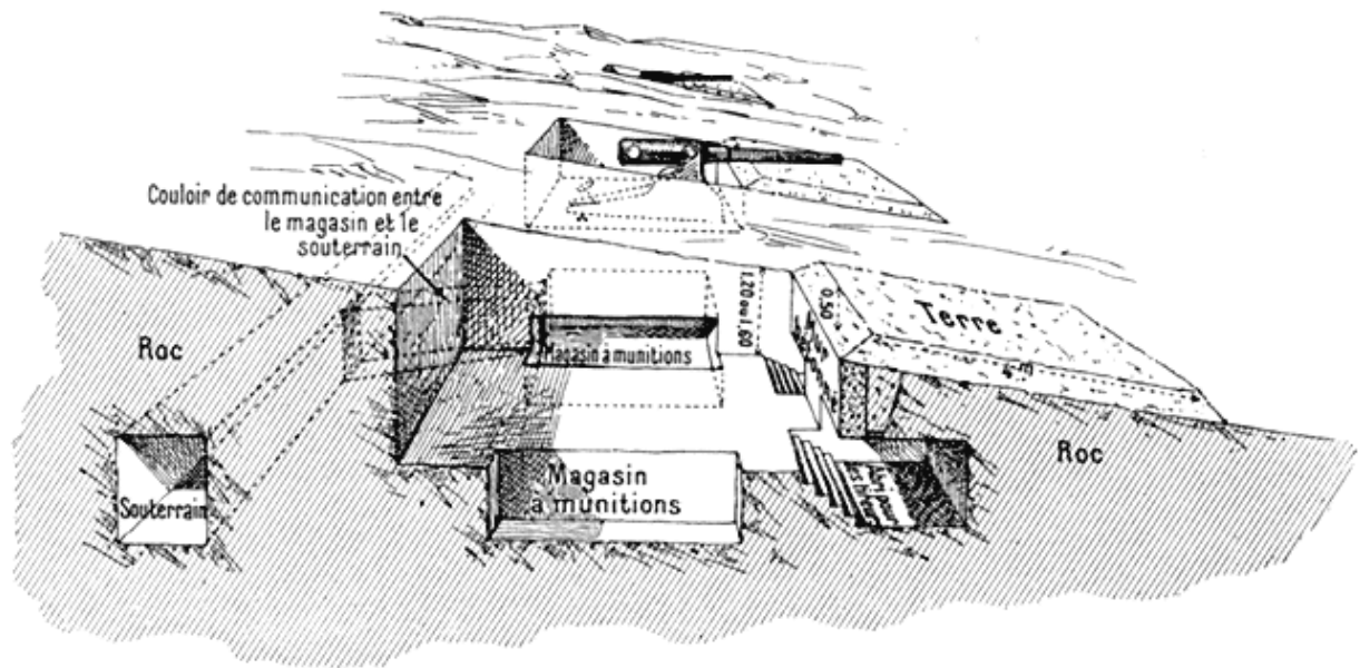
Coupe schématique d'une batterie turque avec ses abris et magasins.
