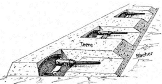
Schéma d'une batterie turque dans laquelle la moitié arrière de chaque emplacement de canon est couverte d'une voûte en béton, elle-même recouverte de terre.
