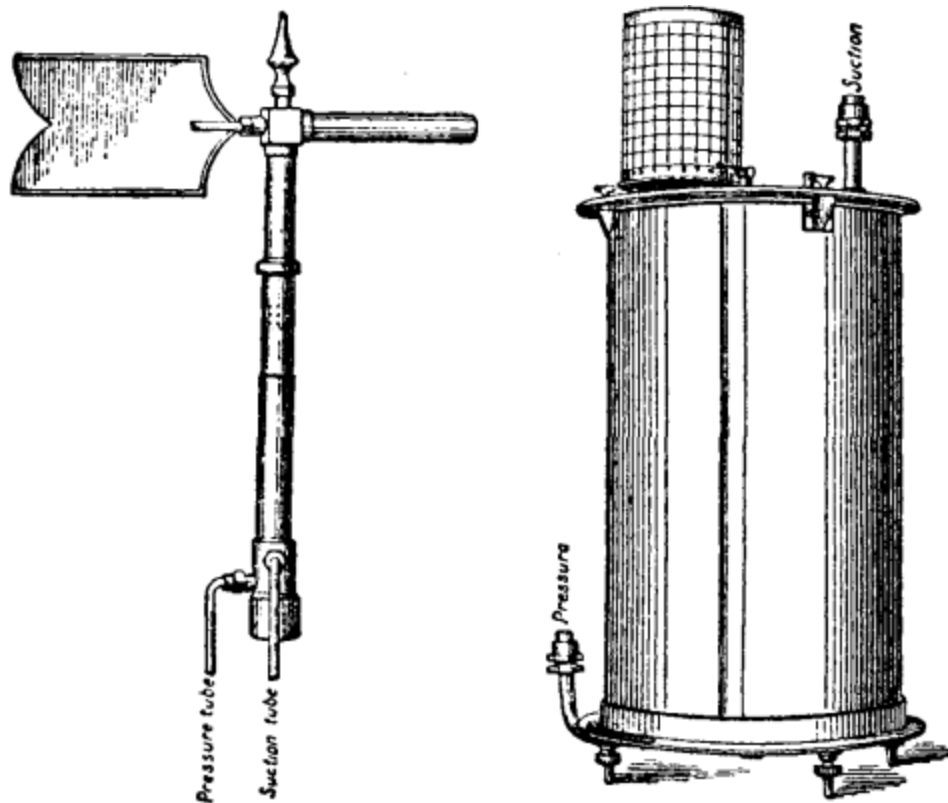
FIG. 1 & FIG. 2 Anemometers.
