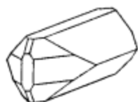
Anglesite specimen.
