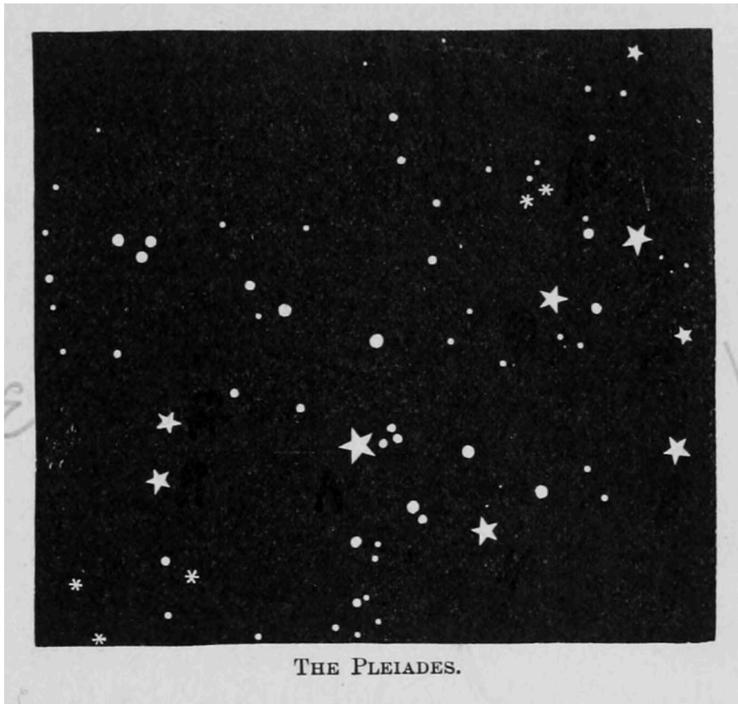
THE PLEIADES.
