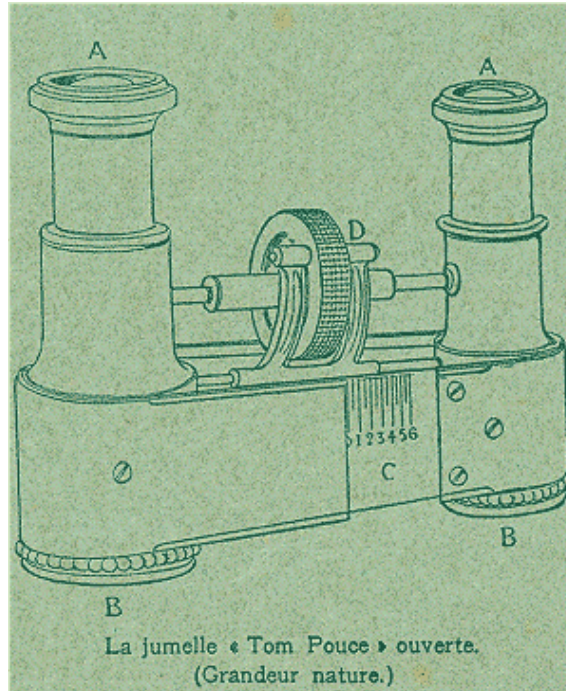
La jumelle «Tom Pouce» ouverte. (Grandeur nature.) AA, oculaires; BB. objectifs; C, traits numérotés indiquant l'écartement des oculaires; D, bielle et mécanisme de mise au point.
