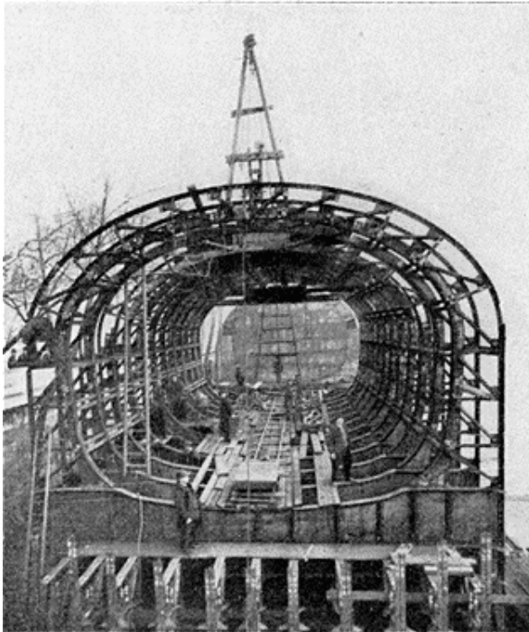
Vue de l'armature métallique des caissons avant l'immersion. Phot. Godefroy.
