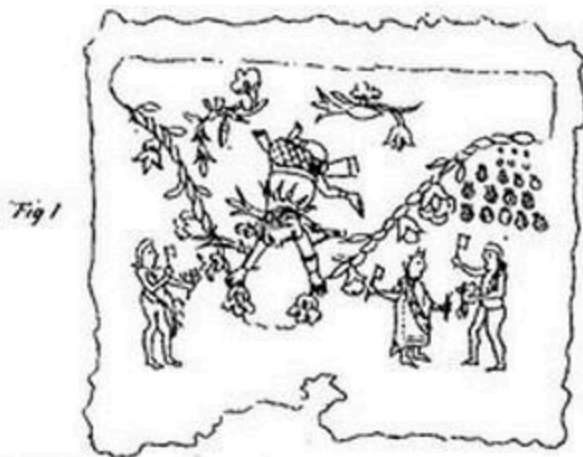
Hiéroglyphes Aztèques conservant le souvenir de quatre époques ou catastrophes de la terre
