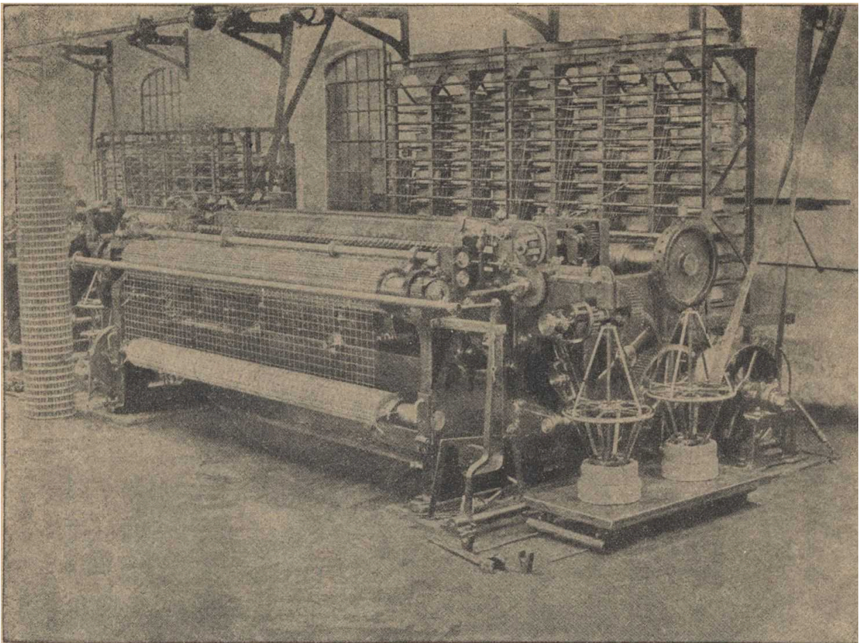
A drótszövő gép
