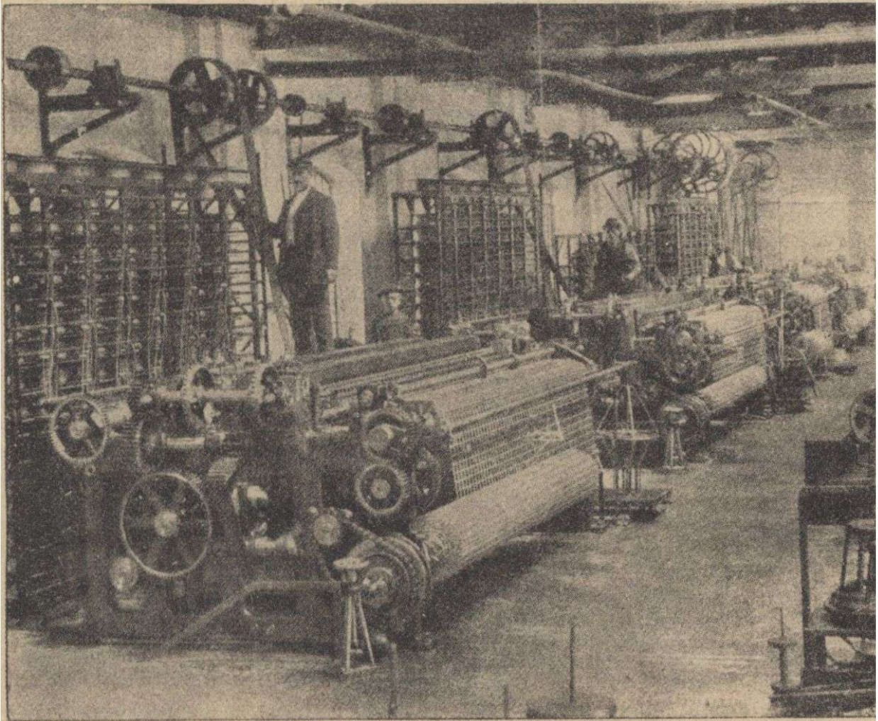
A drótszövő gépek a gyár munkatermében
