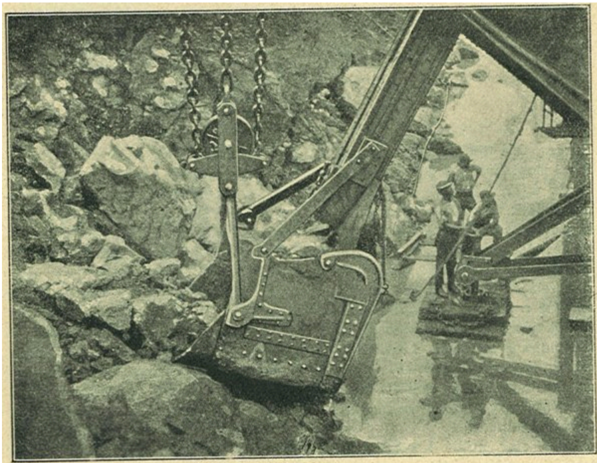
A gőzlapátok munkája
