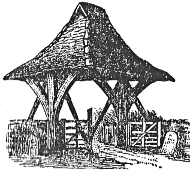
Lichgate.
