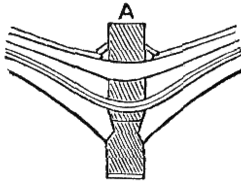
A, Keelson.
