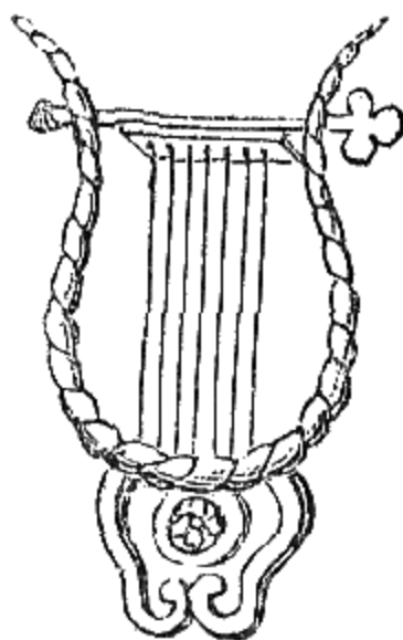
Lyre.
