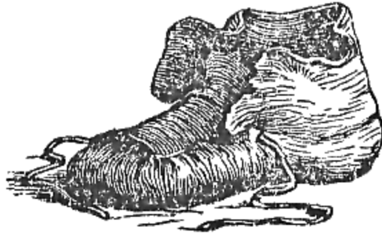
Moccasin.
