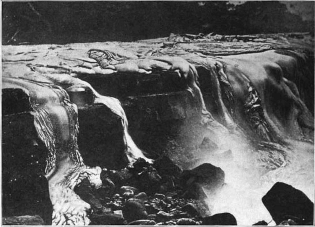
A Lava Cascade.
