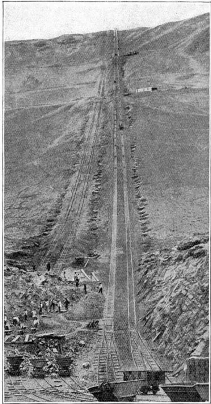
Een kabelspoorweg in een soda-raffinaderij.
