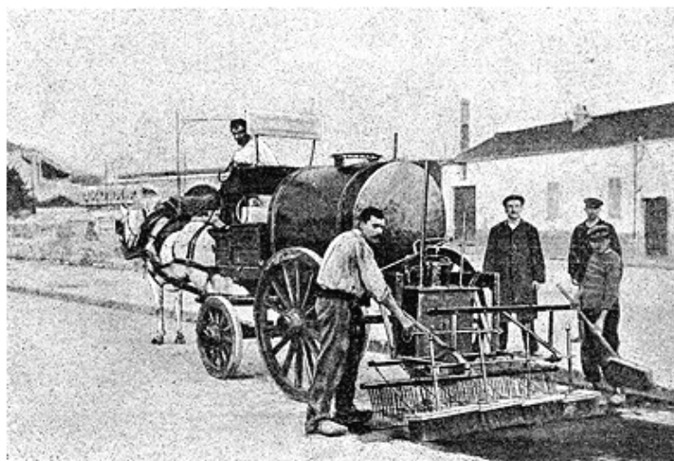
Le tonneau Lassailly, pour le goudronnage automatique des routes.--Phot. de M Martin.
