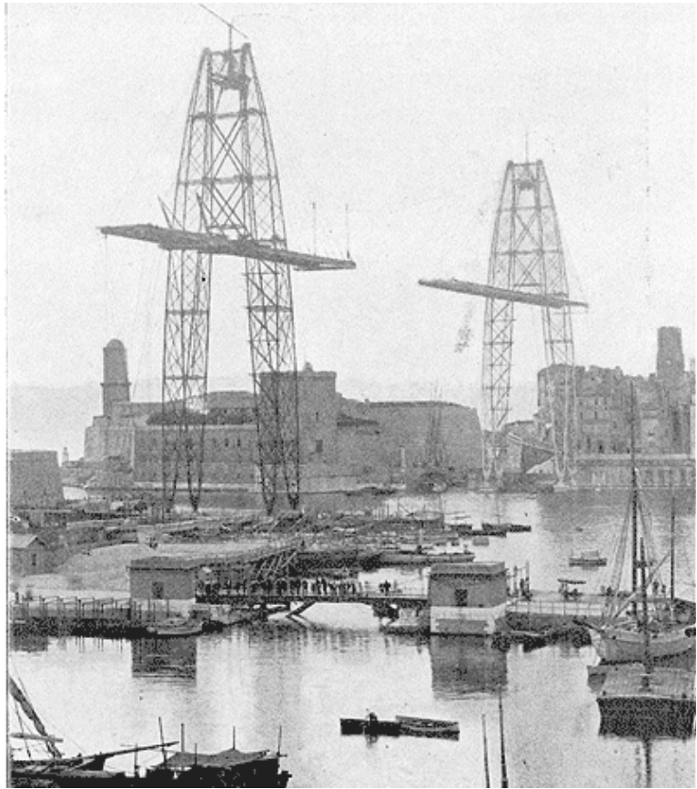
Le nouveau pont à transbordeur de Marseille--Phot. J. Fabre.
