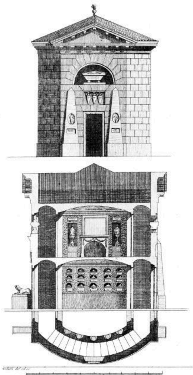
Tav. XXIII. Colombario, ossia cinerario della famiglia degli Acii nel parco di Belgiojoso, con suo spaccato, e pianta.
