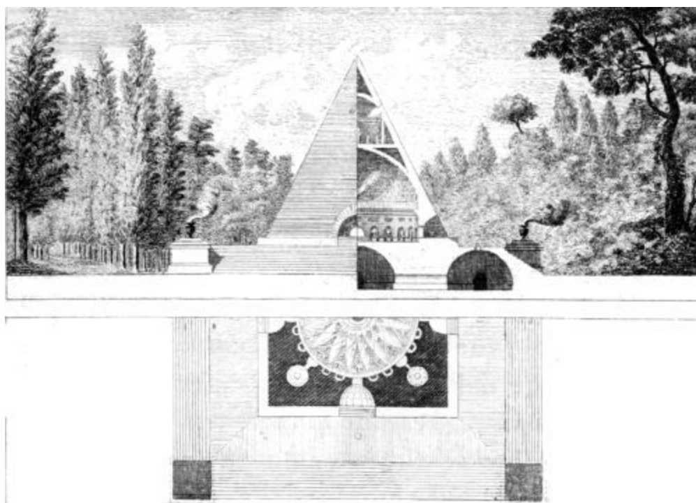
Tav. XXII. Piramide con sua cella, spaccato, e pianta, d'invenzione del cittadino la Gardette.
