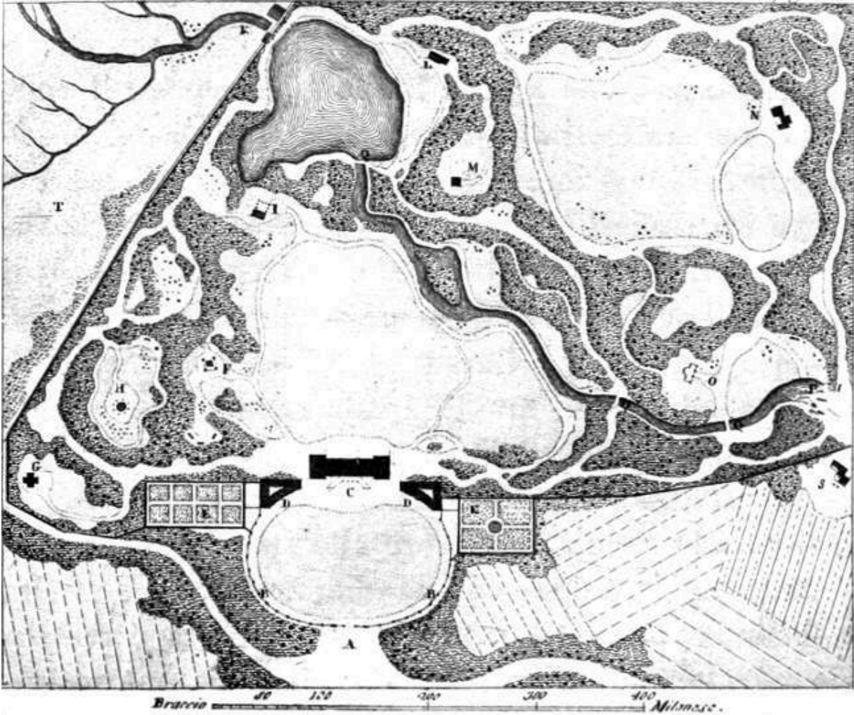
Tav. III. Piano generale di casa, e giardino Inglese.
