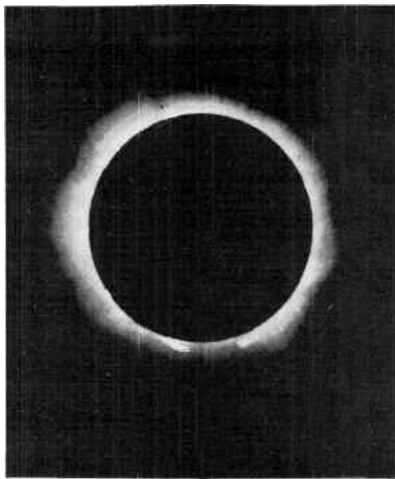
THE SUN'S CORONA.
