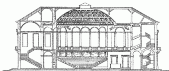
COUPE LATÉRALE.
