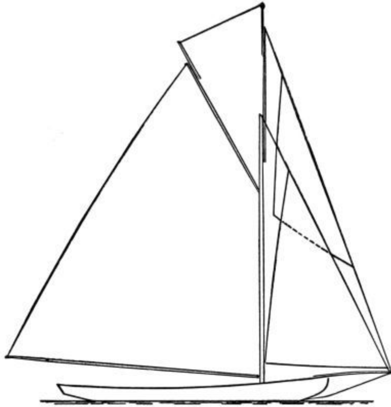
SLOOP RIG
