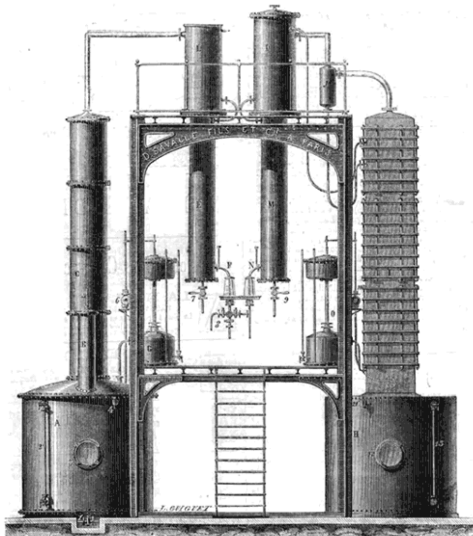
EXPOSITION DE VIENNE.--Les appareils distillatoires de M. Savalle.
