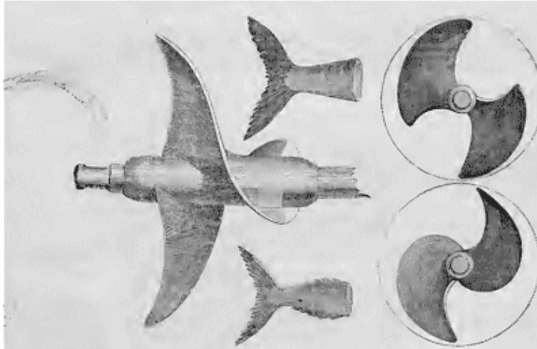
Hélices suivant le système de Rennie.
