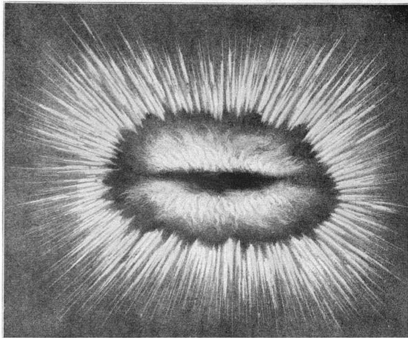
FIG. 5.—AURORAL CORONA.
