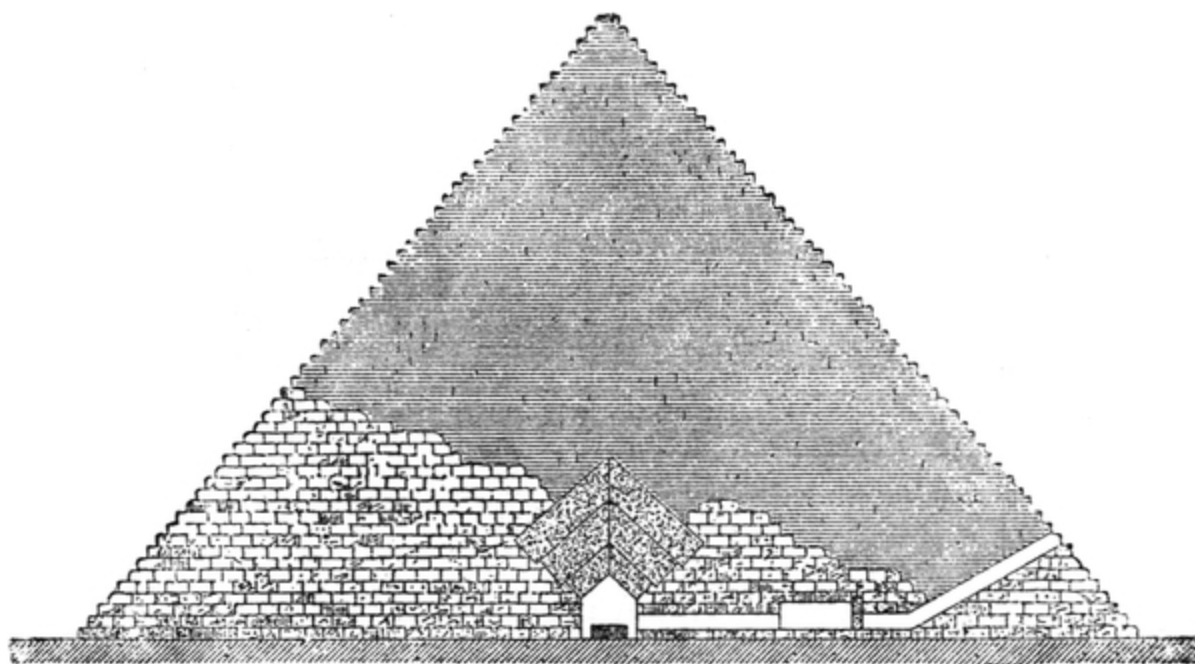
Ein Königsgrab aus dem Alten Reiche. Vertikaldurchschnitt.
