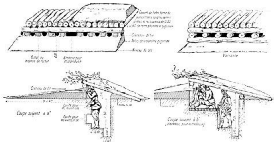
Les tranchées renforcées; détails du couvert, des créneaux et de l'excavation.
