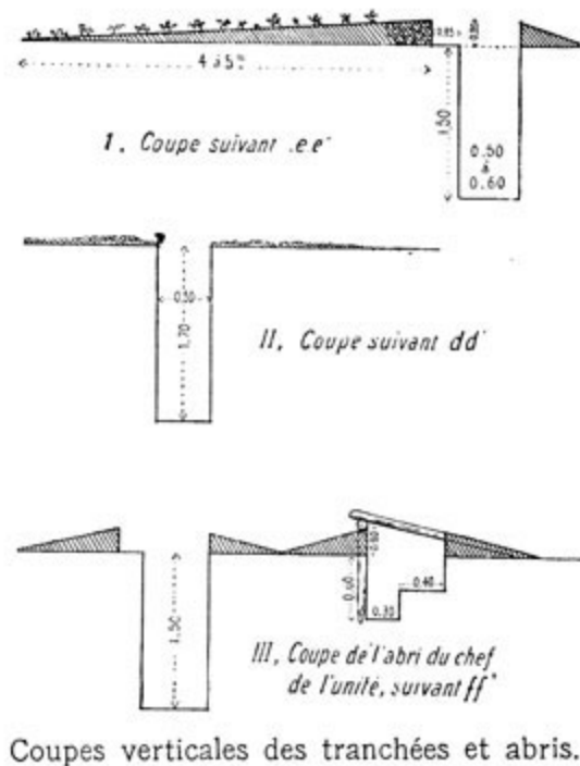
Coupes verticales des tranchées et abris.
