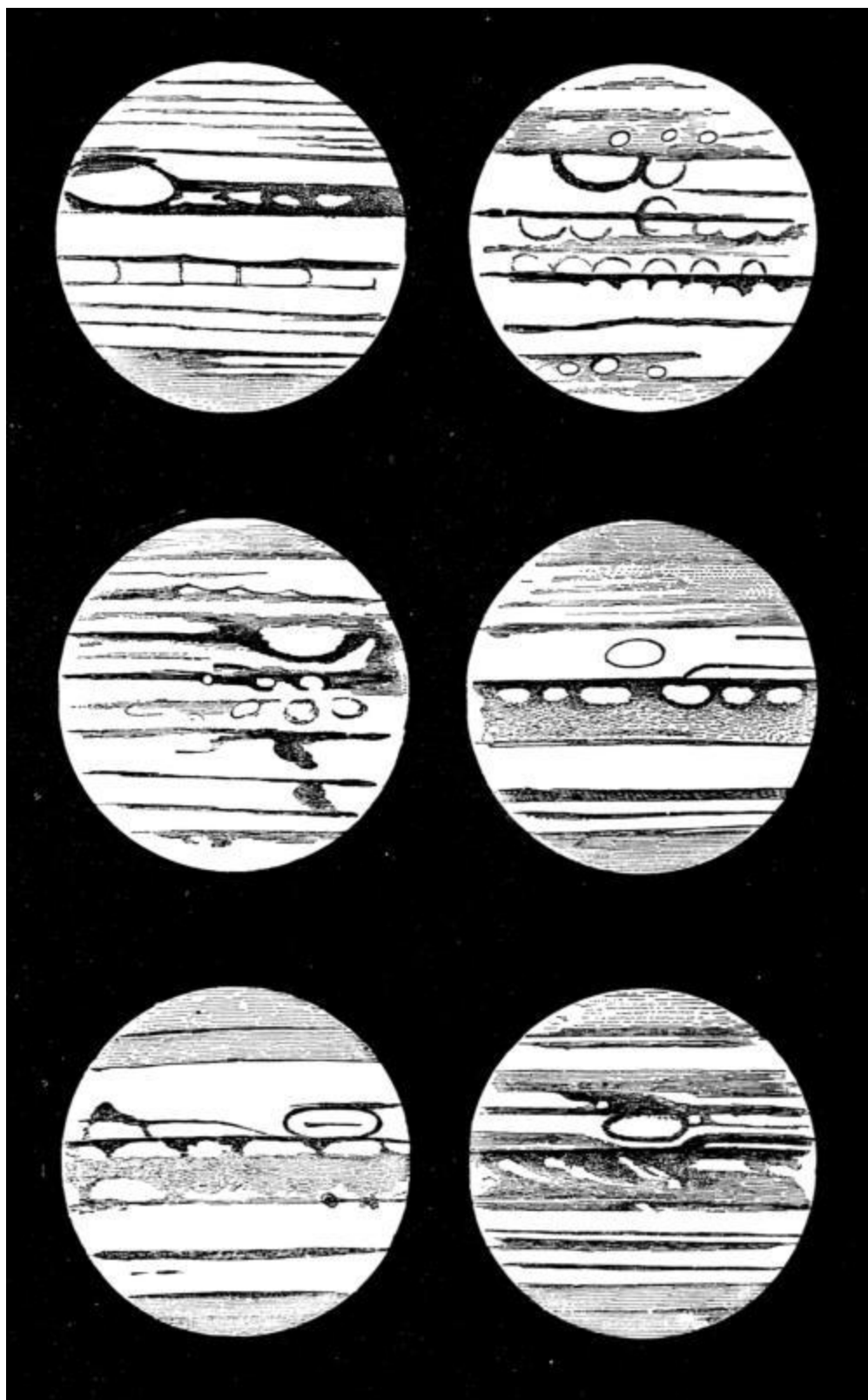
I. 1857, Nov. 27. (Dawes.) III. 1858, Mar. 2. (Huggins.) V. 1872, Feb. 2. (Gledhill.)
