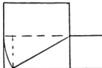
Subtraktion zweier Quadrate.
