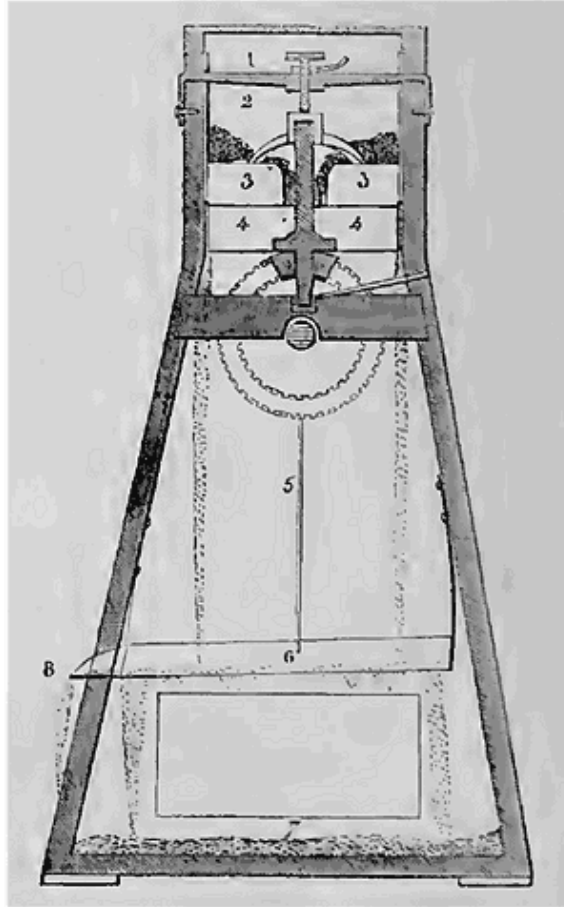
Coupe du Moulin à bras pour l'armée d'Afrique.
