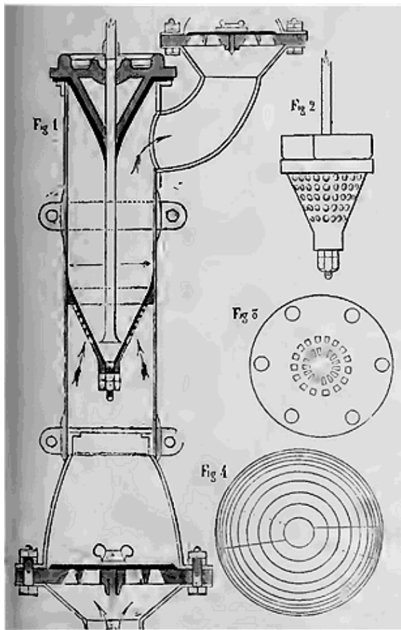
Pompe foulante et aspirante Letestu.
