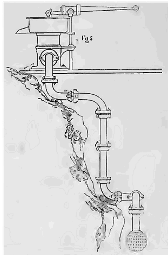
Pompe d'épuisement Letestu, avec la disposition des tuyaux d'aspiration.
