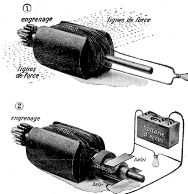
Fig. C.--Induits schématiques--1. Le fil, guipé de coton ou de soie, est bobiné un grand nombre de fois sur une pièce en fer doux, afin que la tension du courant produit soit plus grande; une lampe attachée à ses deux extrémités pourra recevoir ce courant alternatif et s'allumer quand l'induit tournera à une vitesse suffisante.--2. La batterie ne pouvant accepter de courant alternatif, l'induit est muni d'un collecteur qui, au moyen de balais, redresse le courant alternatif; la lampe est ainsi alimentée par du courant continu qui lui vient tantôt de la dynamo, tantôt de la batterie.
