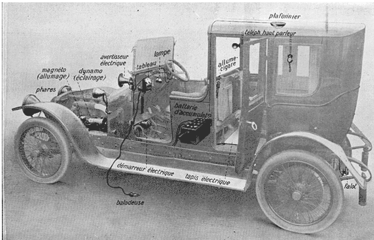
Fig. D.--Les principales applications du courant électrique à bord d'une automobile de 1914.
