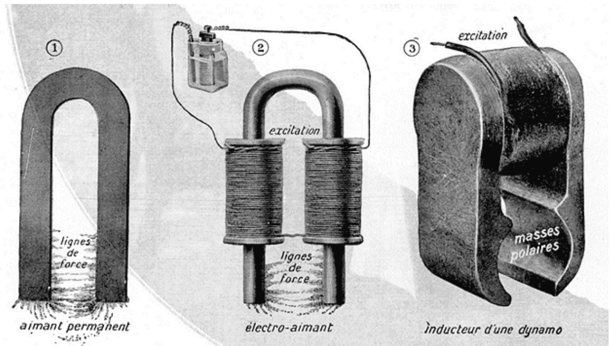
Fig. A.-Aimant permanent et électro aimants.--1. Aimant permanent (morceau d'acier dur recourbé puis aimanté).--2. Electro-aimant (morceau de fer entouré d'une longue spirale qui lui confère les propriétés magnétiques pendant tout le temps qu'elle est traversée par un courant).--3. On donne aux deux extrémités d'un électro-aimant une forme appropriée qu'on nomme masse polaire ; l'ensemble est l' inducteur de la dynamo.
