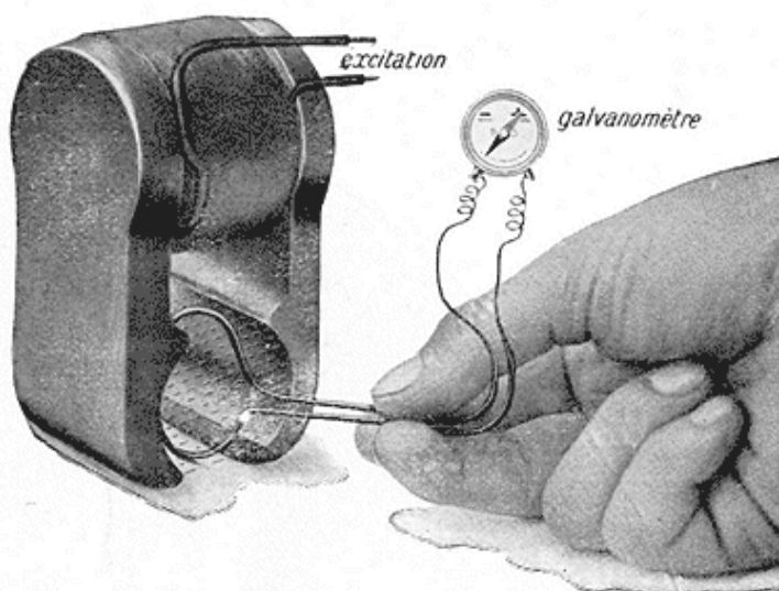
Fig. B.-Expérience schématique montrant qu'un courant est induit dans le fil aux moments où la spire coupe les lignes de force de l'inducteur.
