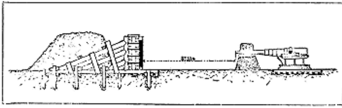
Disposition de la pièce et des cibles.
