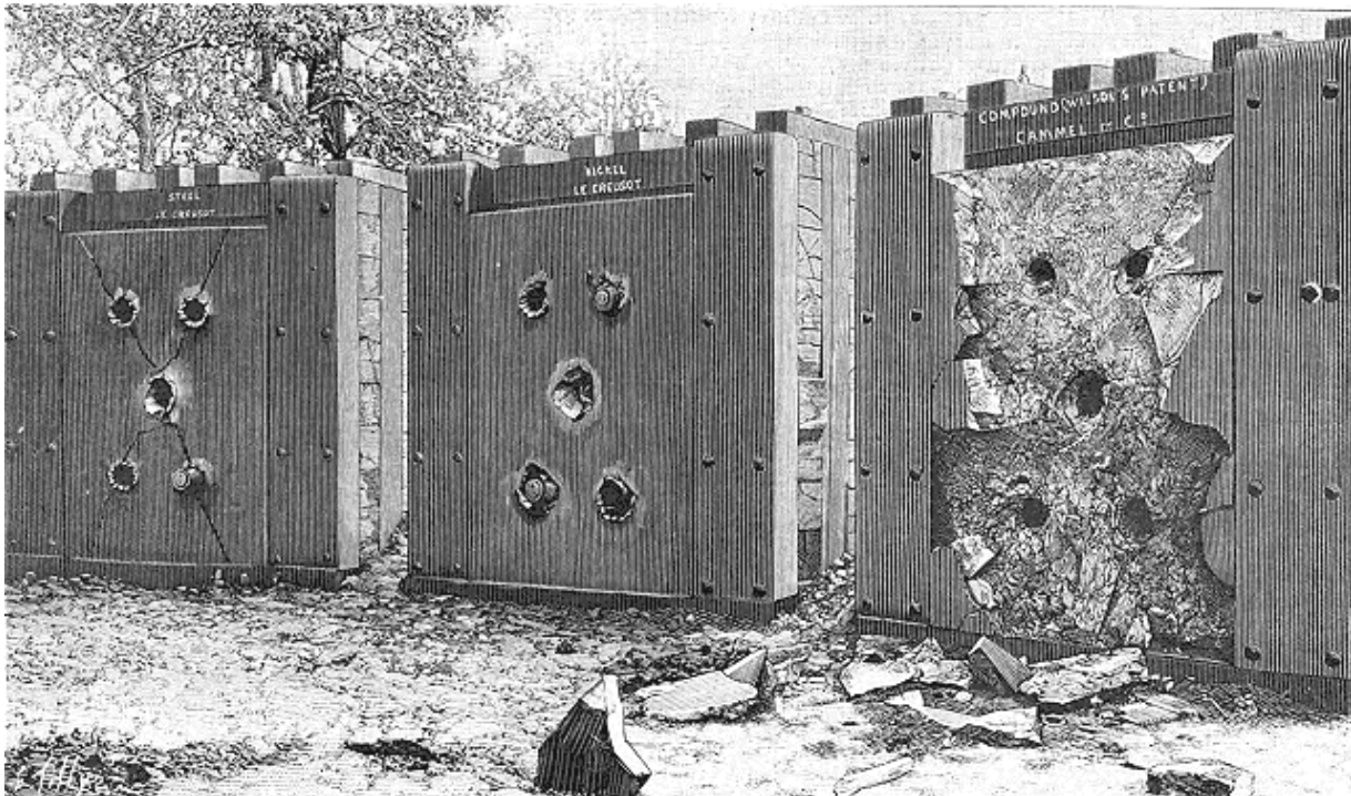
Plaque en acier. Plaque en acier au nickel. Plaque Compound.
