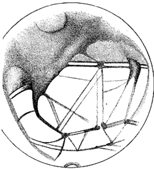
Fig. 5.--Mars en 1890.
