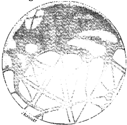
Fig. 5.--Mars en 1890.
