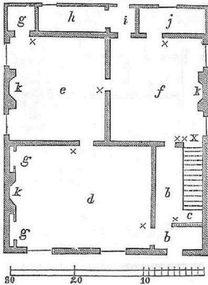
Fig. 27. Ground-plan.
