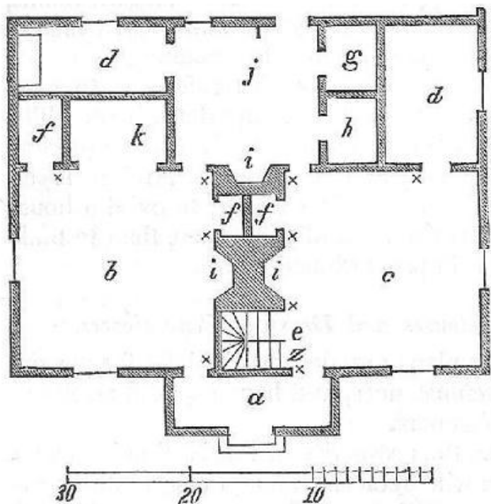
Fig. 18. Ground-plan.
