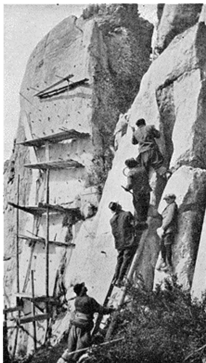
Les échafaudages dressés pour le percement des 237 trous de mine.
