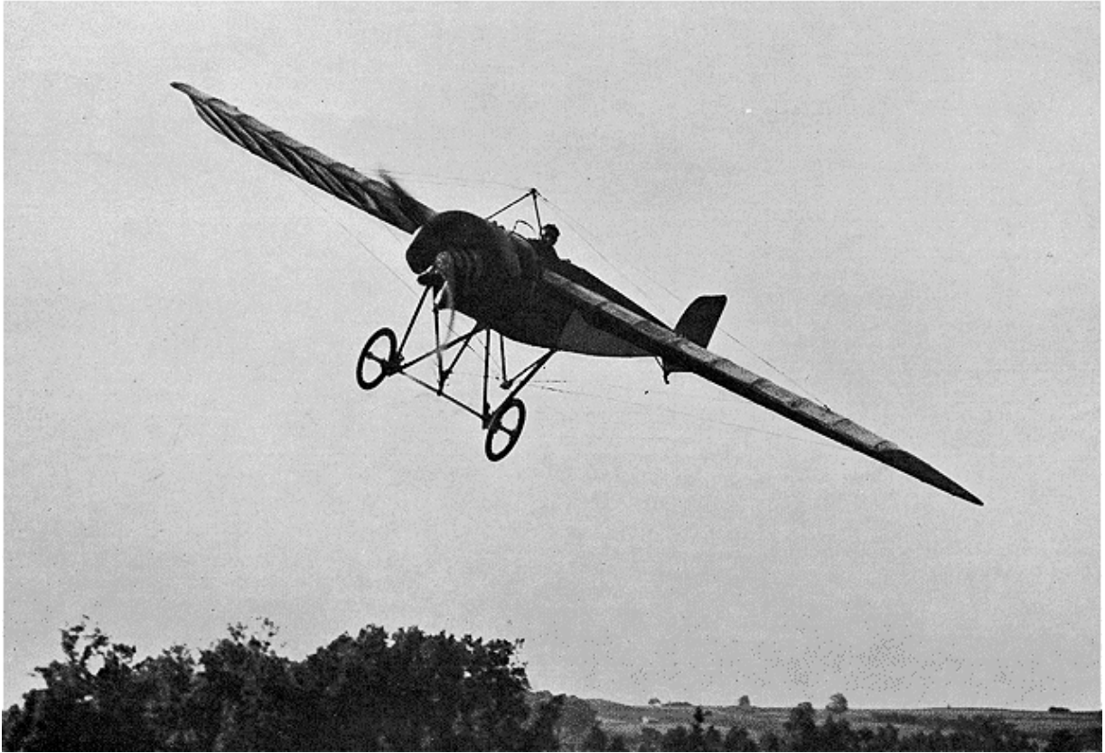
Audemars virant à sept mètres du sol. Le monoplane étant à peu de distance de l'opérateur, l'objectif a nettement enregistré la manoeuvre du gauchissement de l'aile. --Phot. Bergeron.
