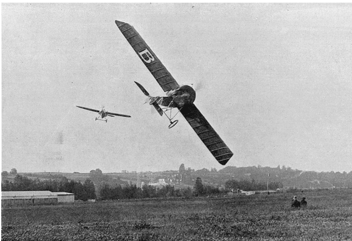
La poursuite : Brindejone des Moulinais, suivi par Guillaux.--Phot. Bracher.
