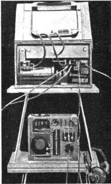
Geber und Empfänger einer modernen Telefunken-Station.
