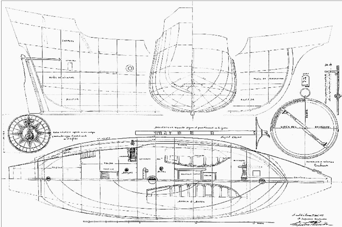
PLANO DE TRAZADO
