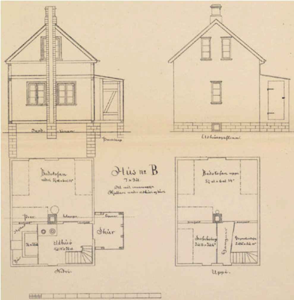
Hús B - 7×9 álnir
