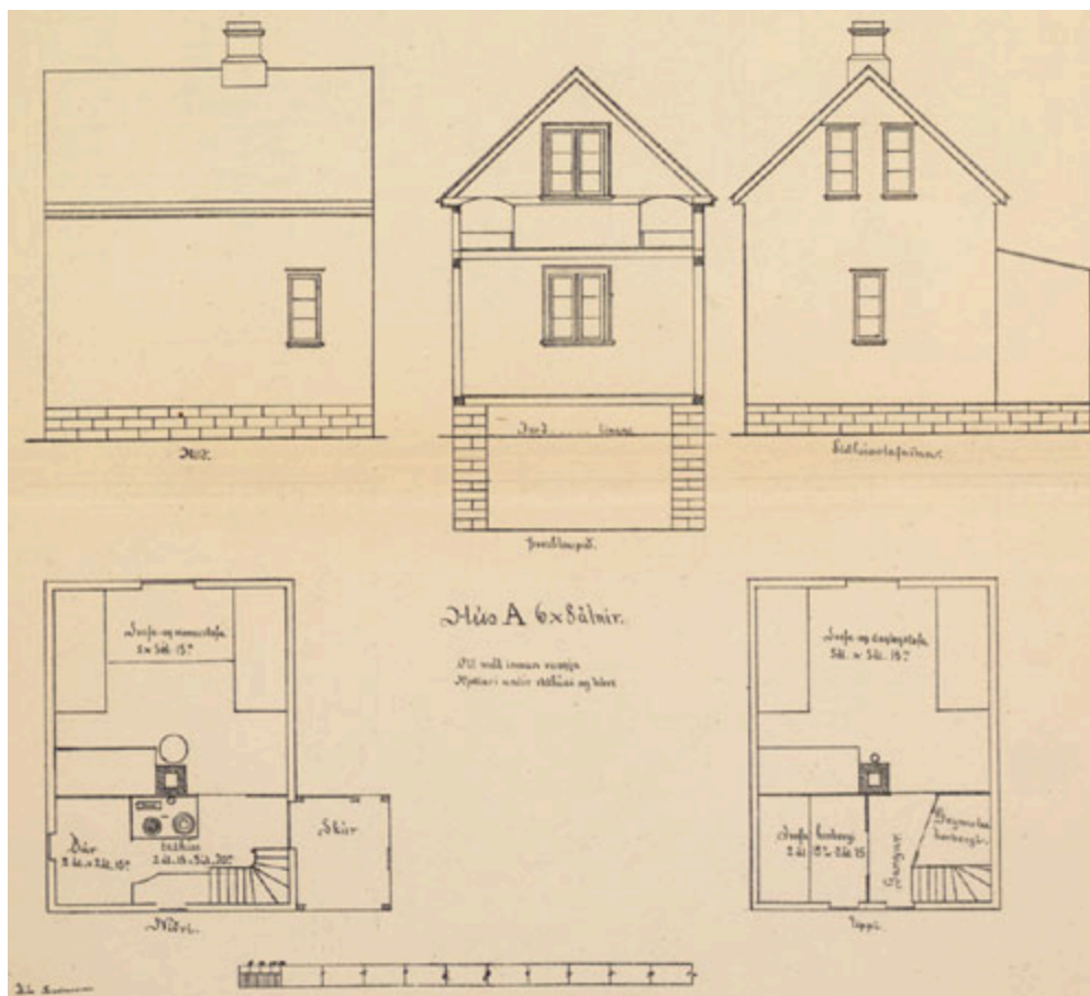
Hús A - 6×8 álnir
