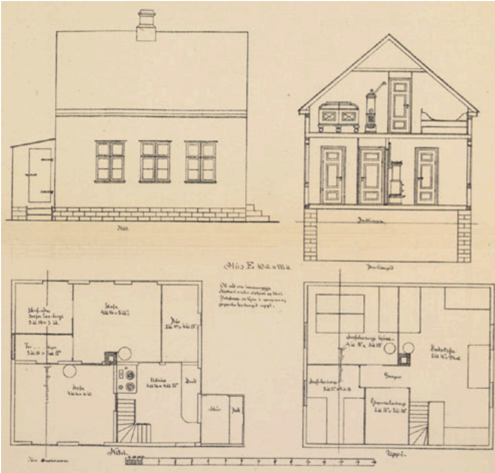
Hús E - 10×11½ álnir
