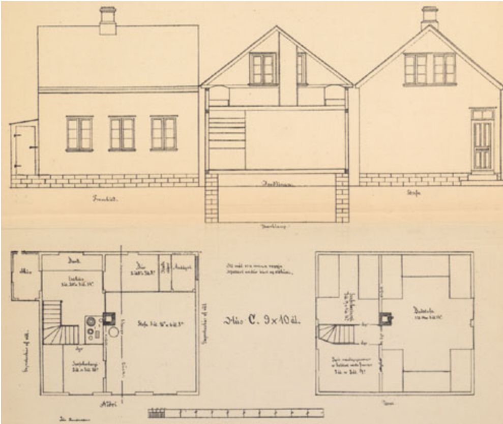
Hús C - 9×10 álnir
