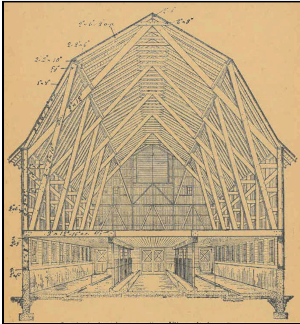
Standard-rakenteinen navetta. Ylinen itsekannattava.
