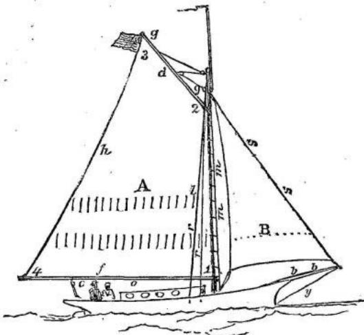
SLOOP.
