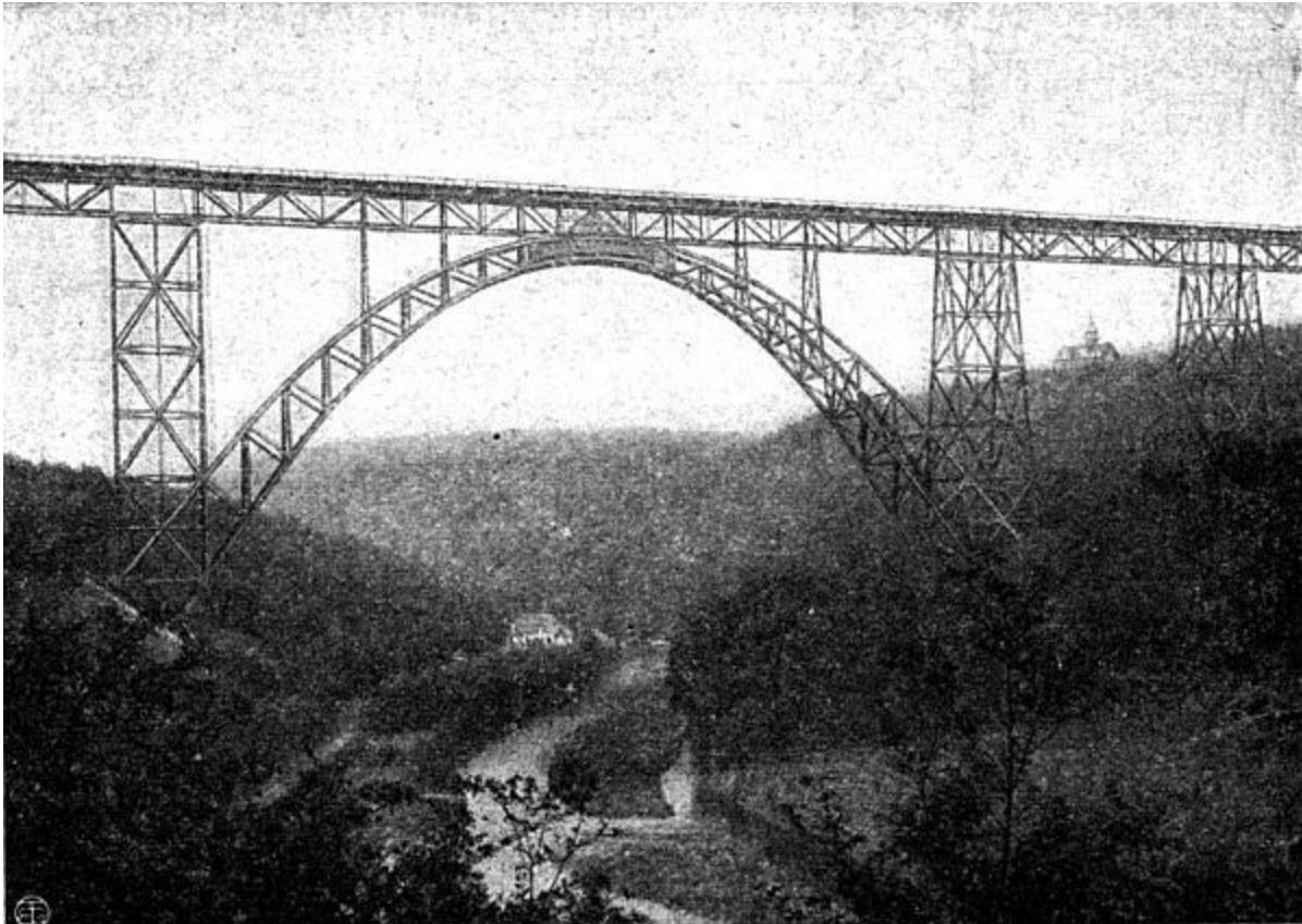
Abb. 1. Die Wupperbrücke bei Müngsten.
