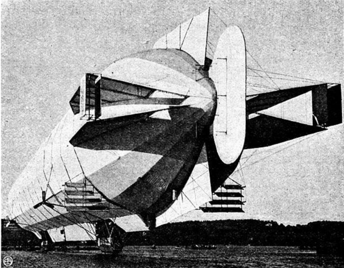
Abb. 27. Die Steuereinrichtung des Zeppelin-Luftschiffes.
