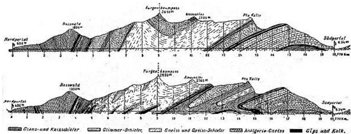
Abb. 10. Das Profil des Simplonmassivs.
