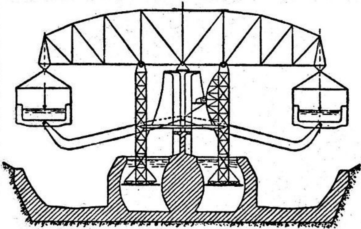
Abb. 13. Das projektierte Schiffshebewerk bei Nieder-Finow.
