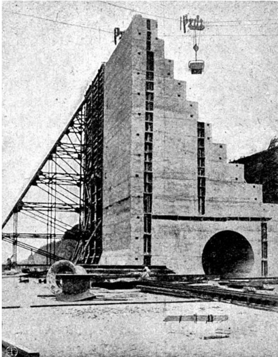
Abb. 12. Eine Schleuse des Panama-Kanals im Bau.
