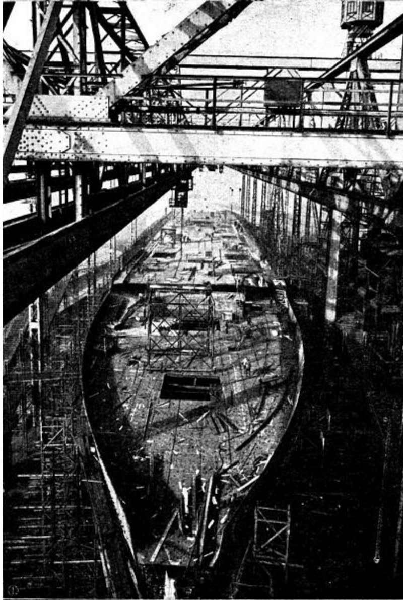
Abb. 25. Der Turbinen-Schnelldampfer »Vaterland« der »Hapag« im Bau.
