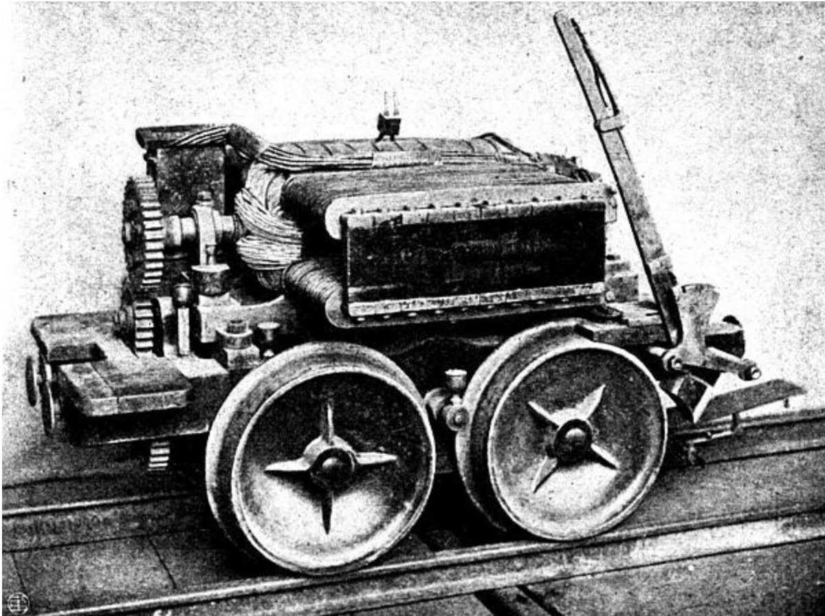
Abb. 16. Die erste elektrische Lokomotive. 1879.
