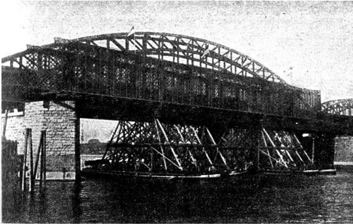
Abb. 5. Das Ausfahren der alten Rheinbrücke bei Köln.
