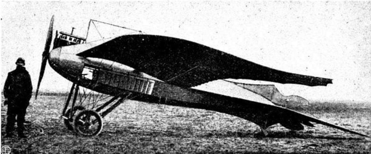
Abb. 30. Rumpler-Eindecker.
