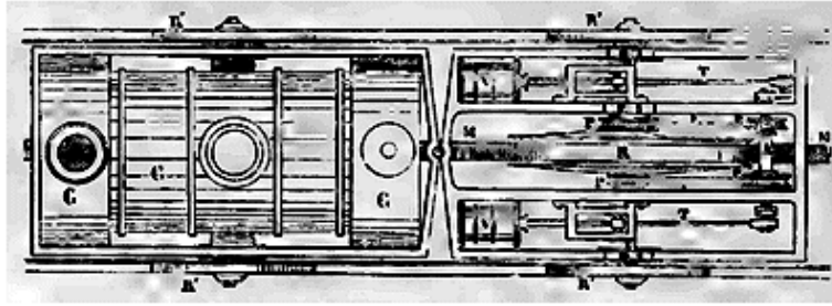
Fig. 2.--Plan de la locomotive.
