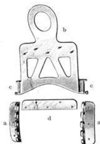
Fig. 32. Schnellsattler.
