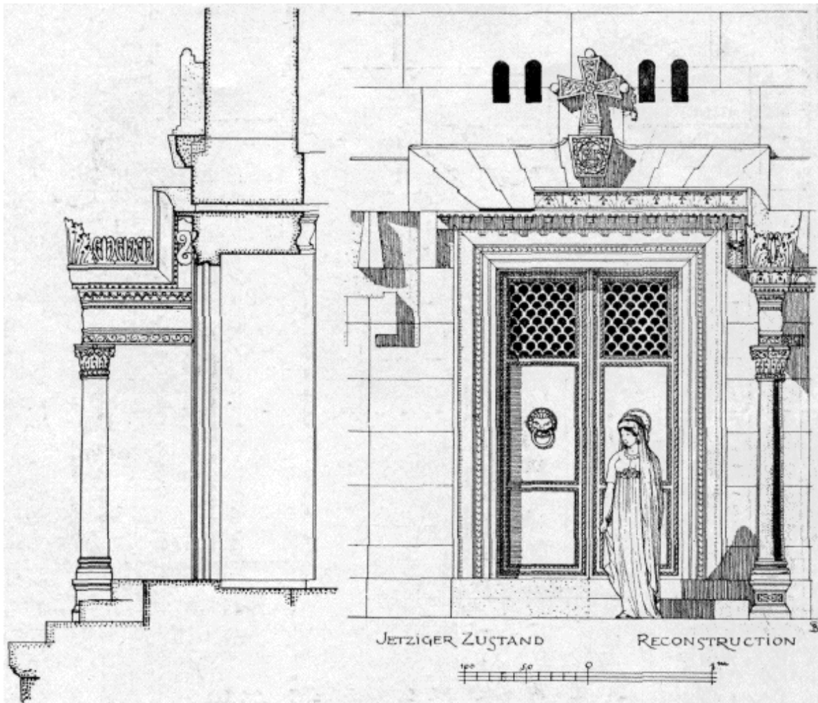
Bild 22. Die Türwand des Obergeschosses.
