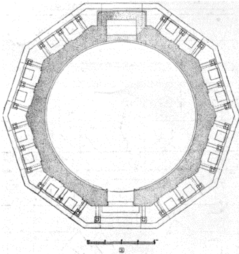
Bild 24. Grundriss des Obergeschosses, rekonstruiert von Bruno Schulz.
