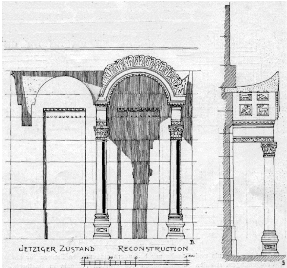
Bild 15. Die acht gleichen Wände des Obergeschosses.
