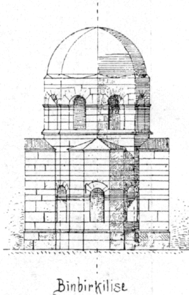
Bild 32. Centralbau von Binbirkilise nach Darstellung Durms.
