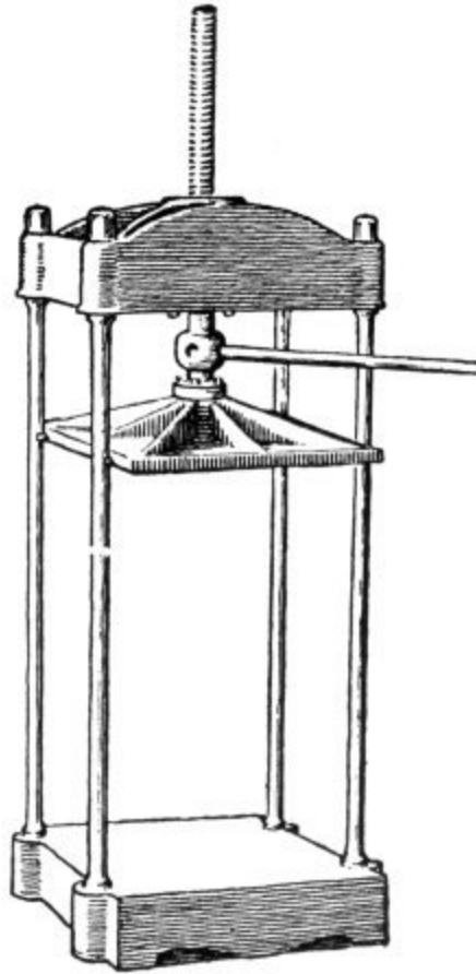
Fig. 21.—Standing Press
