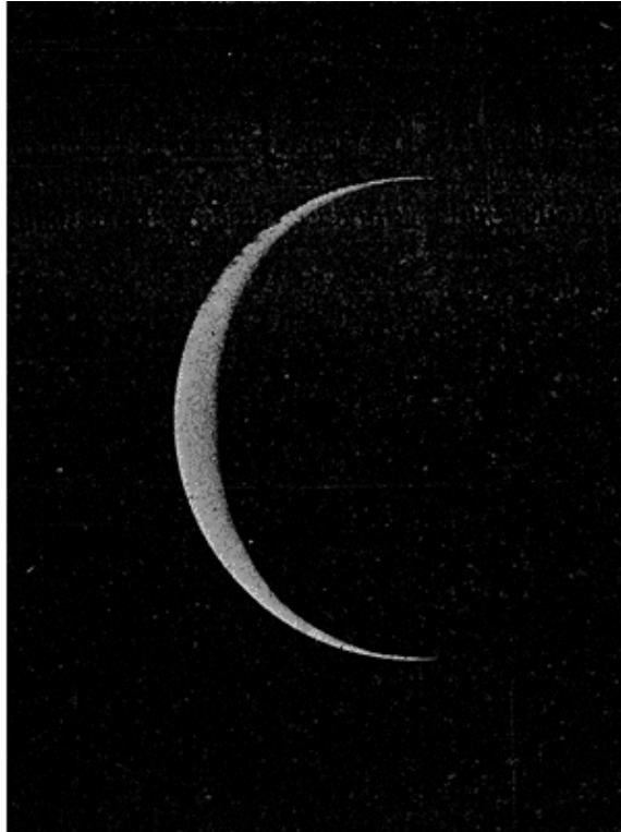
Aspect télescopique actuel de la planète Vénus. (Observatoire de Juvisy.)
