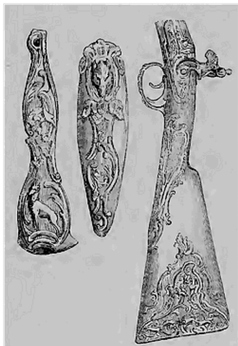
Fusil style Louis XV, exécuté par M. Caron.--Aspect de la crosse et développement du porte-baguettes et du dessous de crosse.
