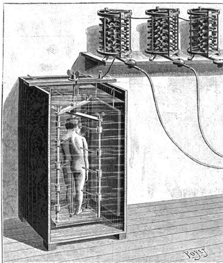
Immersion du sujet dans le bain galvanique.
