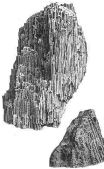
Versteinertes Holz aus der Ammons Oase.
