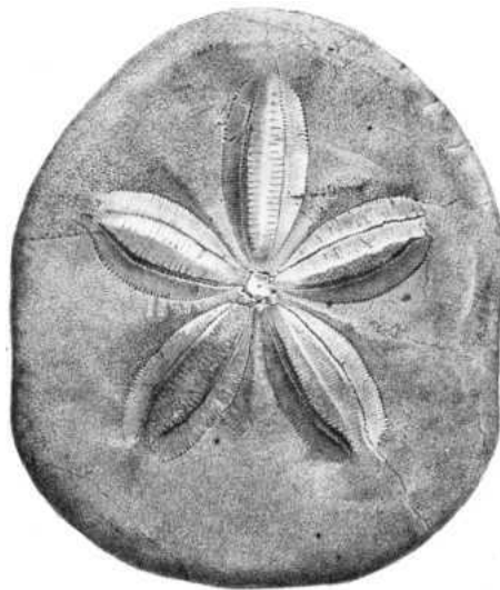
Asterit aus der Oase des Jupiter-Ammon.
