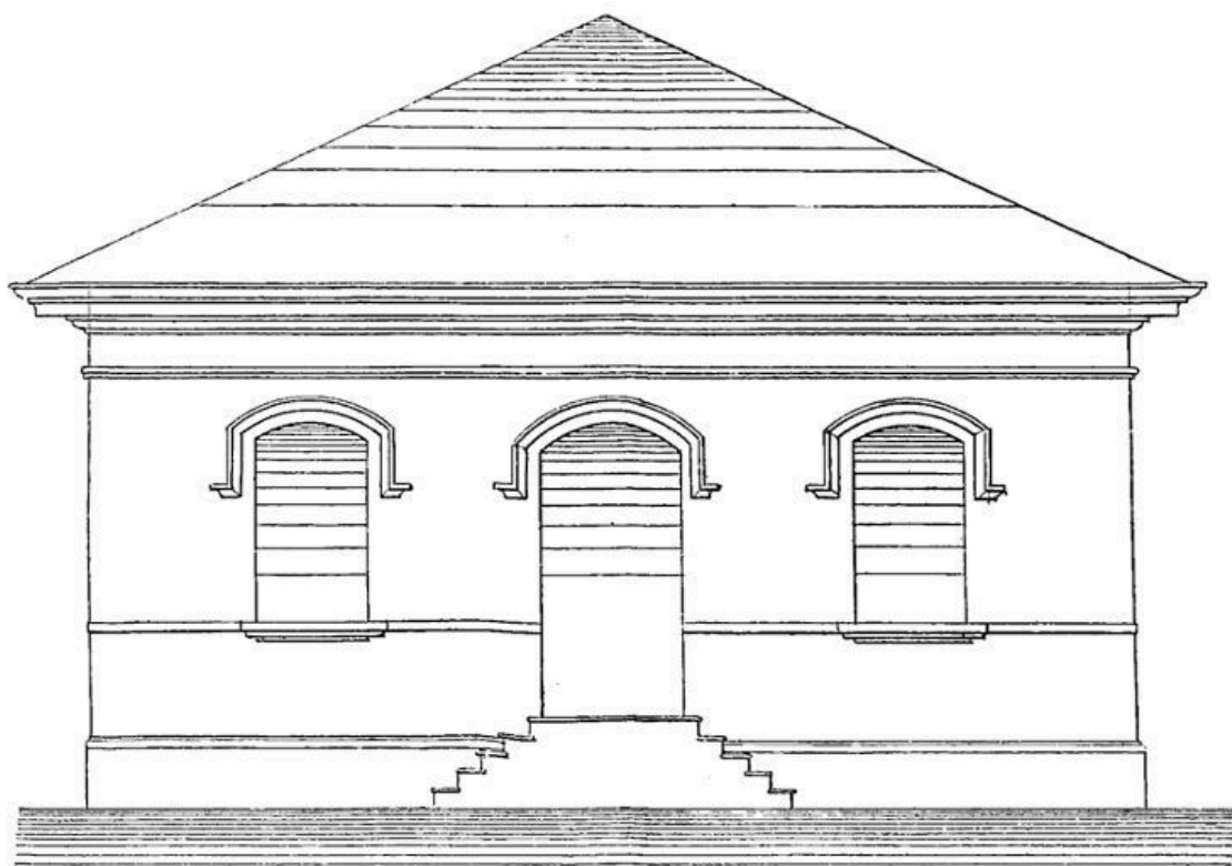
TAVOLA I. Fig. 3 — PROSPETTO — Facciata a sud. (Scala 1:100). Ing. B. FOLLI, dis.
