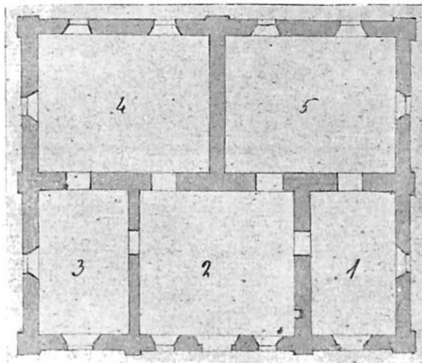
Fig. 2. PIANTA: 1. Vestibolo. — 2. Cucina. — 3. Salatoio — 4. Casera — 5. Deposito latte.
