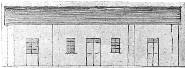
Fig. 1. PROSPETTO: — Fabbricato per una latteria sociale — Scala 1 : 200.
