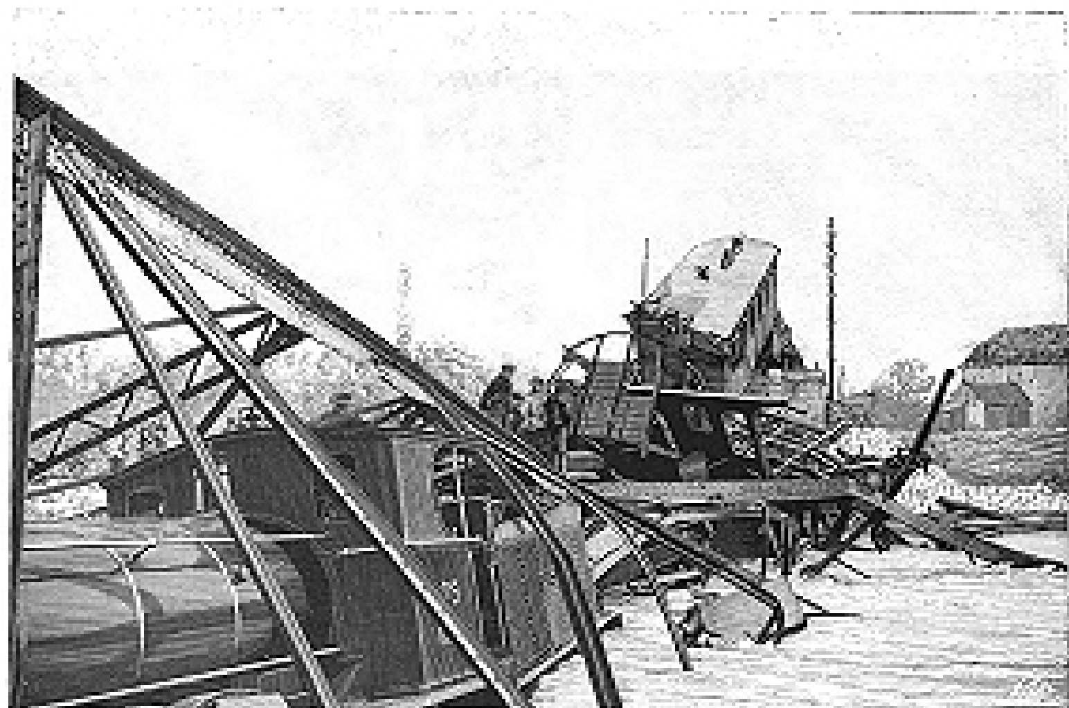
LA CATASTROPHE DE MICHENHEIM. — Les machines renversées par la dégrè. — Photographie Yvels.
