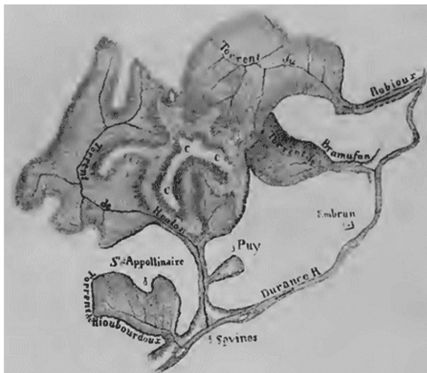
Torrents.--Plan de la vallée de la Durance.
